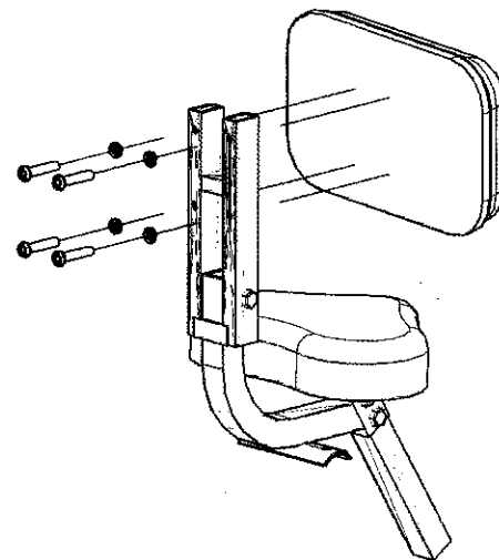
4.背もたれの取付け
