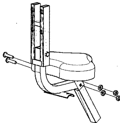
3.背もたれネックの取付け
