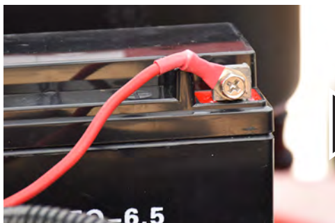
必ず赤いコードから接続します。 +に接続します。
